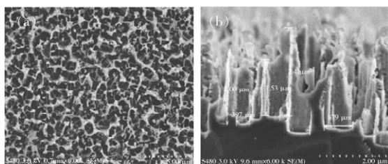
图 1 离子注入后硅片表面的表面形貌。(a) 俯视图图像; (b) 截面图像。
