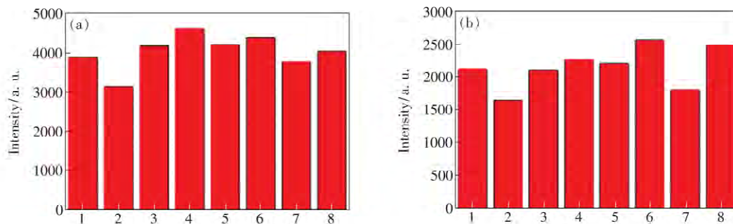
图 9 相同衬底的 8 个位置上两个特征峰的信号强度。(a) 614\text{ cm}^{-1} ; (b) 1650\text{ cm}^{-1} 。
