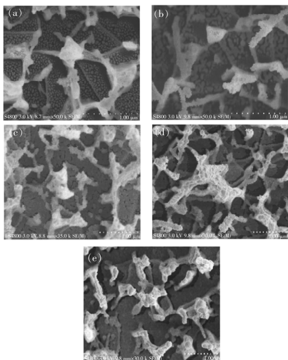
图 3 不同镀银厚度衬底表面形貌的俯视图。(a) 10 nm; (b) 30 nm; (c) 40 nm; (d) 50 nm; (e) 80 nm。
