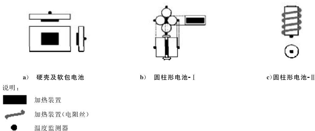
图 C.2 加热触发时温度传感器的布置位置示意图
