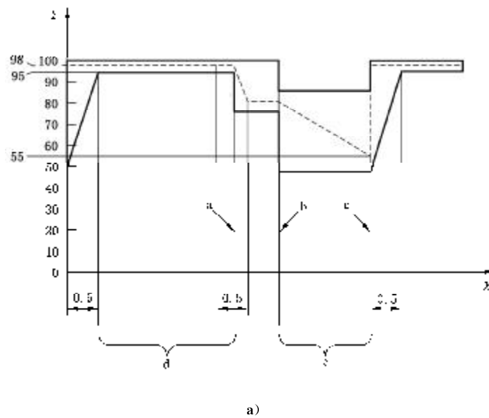
图 8 温湿度循环
