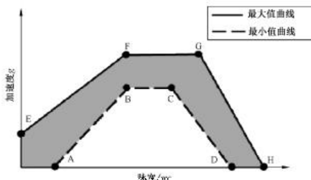
图5 模拟碰撞脉冲容差范围示意图
